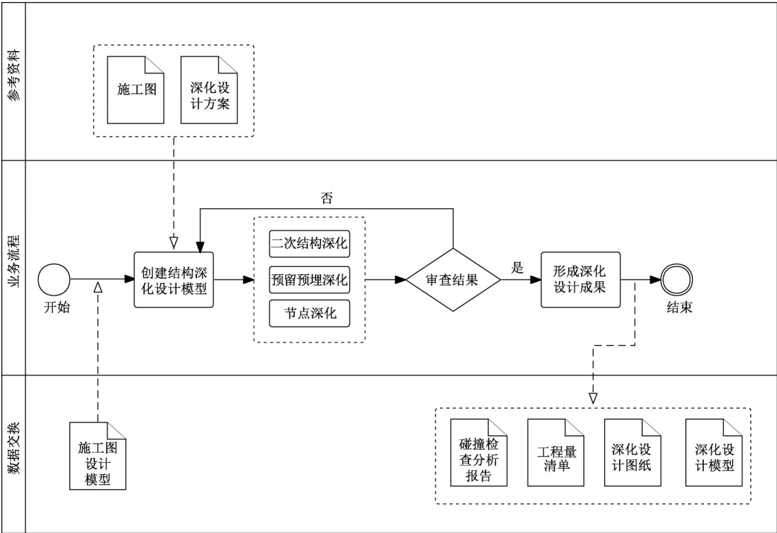
图2 现浇混凝土结构深化设计BIM应用流程
