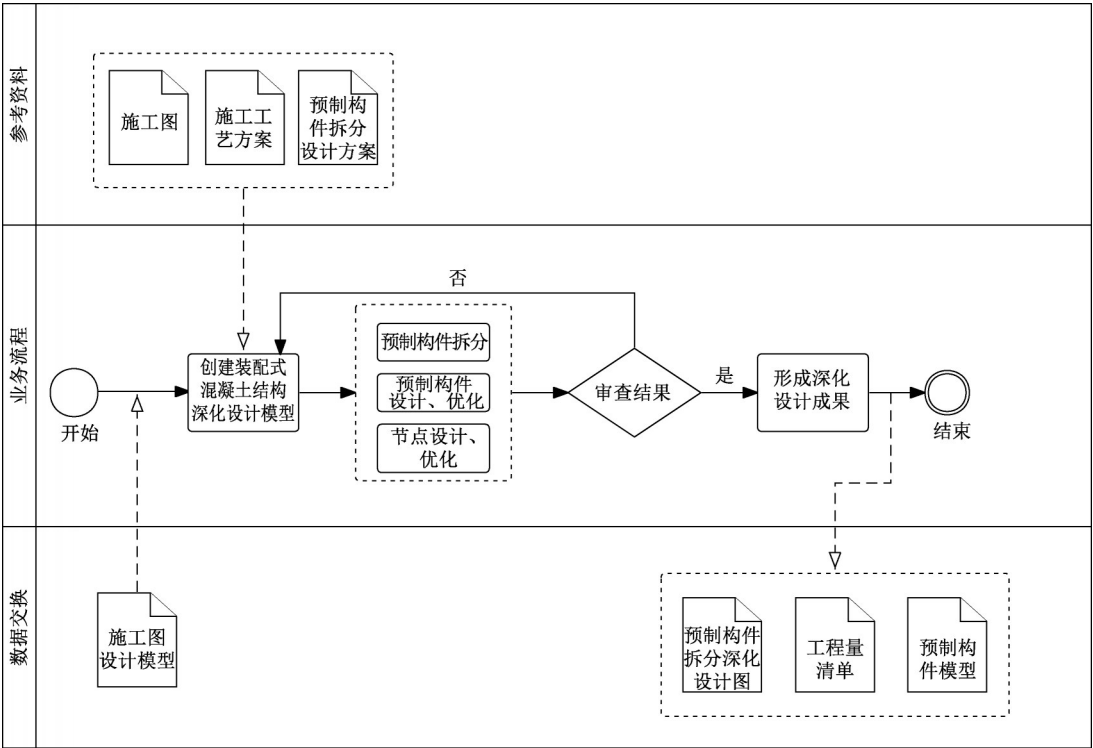
图3 装配式混凝土结构深化设计BIM应用流程
