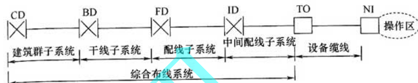
图 3.7.3 工业环境布线系统架构
