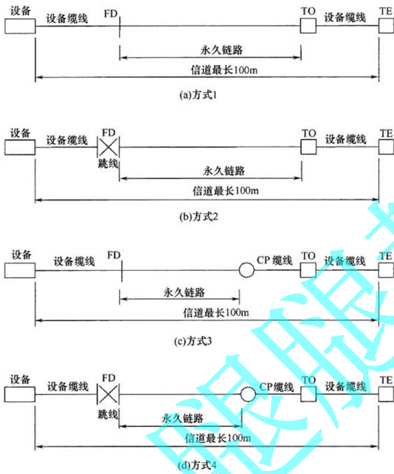
图 3.3.3-1 配线子系统信道连接方式
