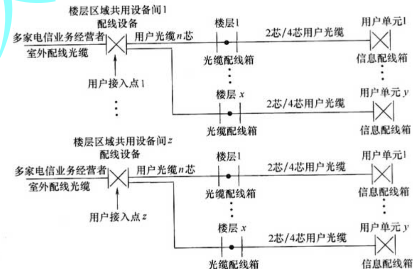
图 4.2.2-2 用户接入点设于建筑物楼层区域共用设备间
