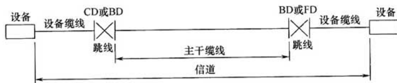
图 3.3.3-2 干线子系统信道连接方式
