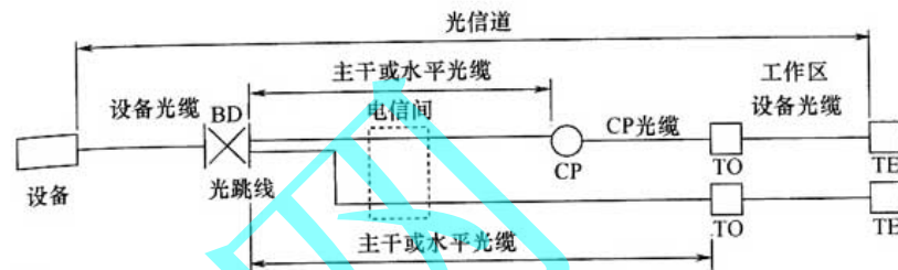
图 3.2.4-3 光纤信道构成 3
