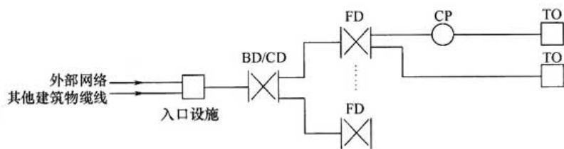
图 3.1.2-3 综合布线系统引入部分构成
