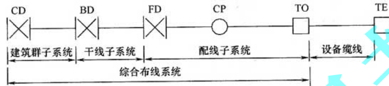
图 3.1.2-1 综合布线系统基本构成
