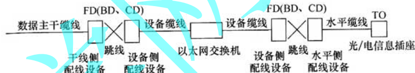
图 5.2.3-2 交叉连接方式
