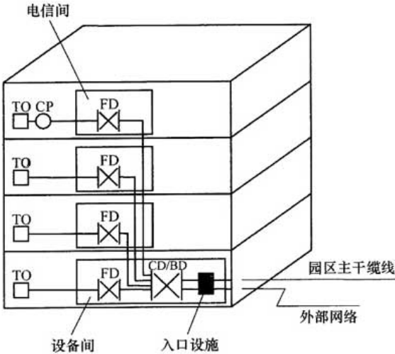
图 1 综合布线配线设备典型设置
