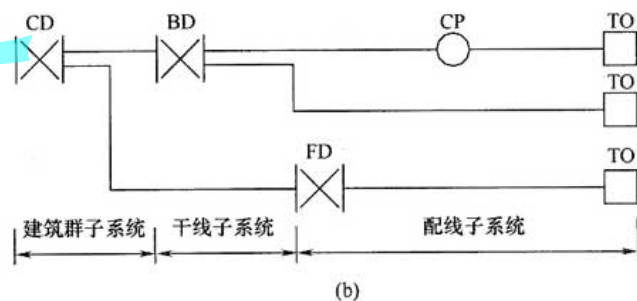
图 3.1.2-2 综合布线子系统构成
