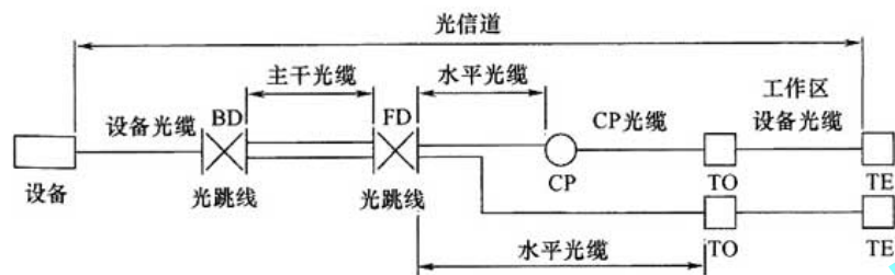
图 3.2.4-1 光纤信道构成 1
