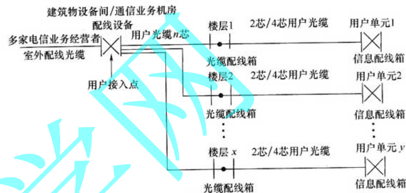
图 4.2.2-1 用户接入点设于单栋建筑物内设备间
