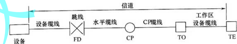
图 3.3.2 配线子系统缆线划分
