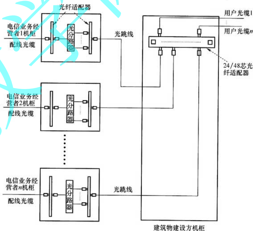
图例: □ 光纤连接器 (SC/FC/LC)
