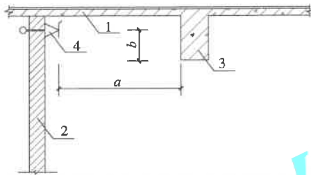
图 7.2.6 边墙型洒水喷头与正前方障碍物的距离 1—顶板;2—背墙;3—梁(或通风管道);4—边墙型喷头
